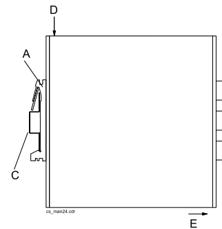
Abb. 2.4.2: CS Demontage
