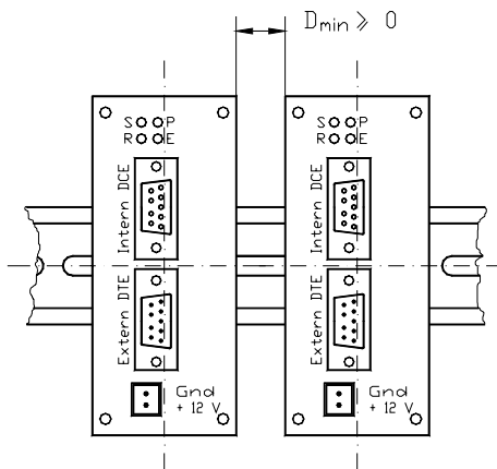
Abb. 2.4.1: FWU-Anordnung
