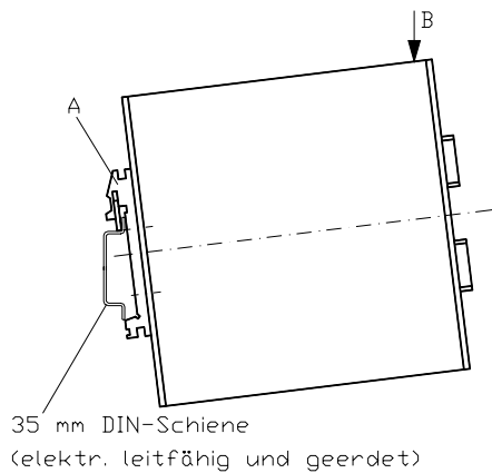
Abb. 2.4.2: FWU-Montage
