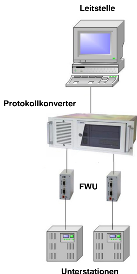
Abb. 2.1: Prinzipieller Aufbau Leitwarte – Protokollkonverter FWU - Unterstation
