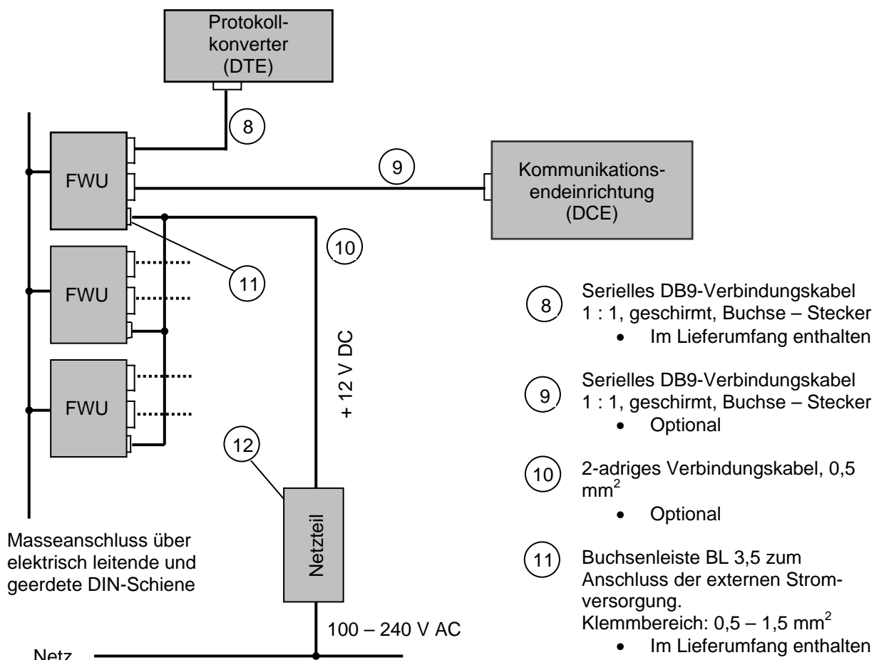
Abb. 2.5.1: Elektrische Installation
