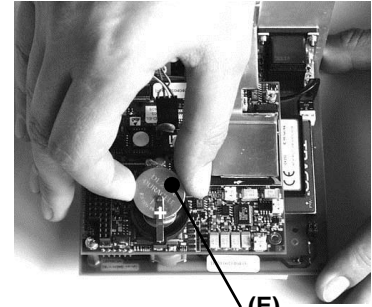
Abb. 2.5.6 Austausch der Batterie (E). Polung beachten.
