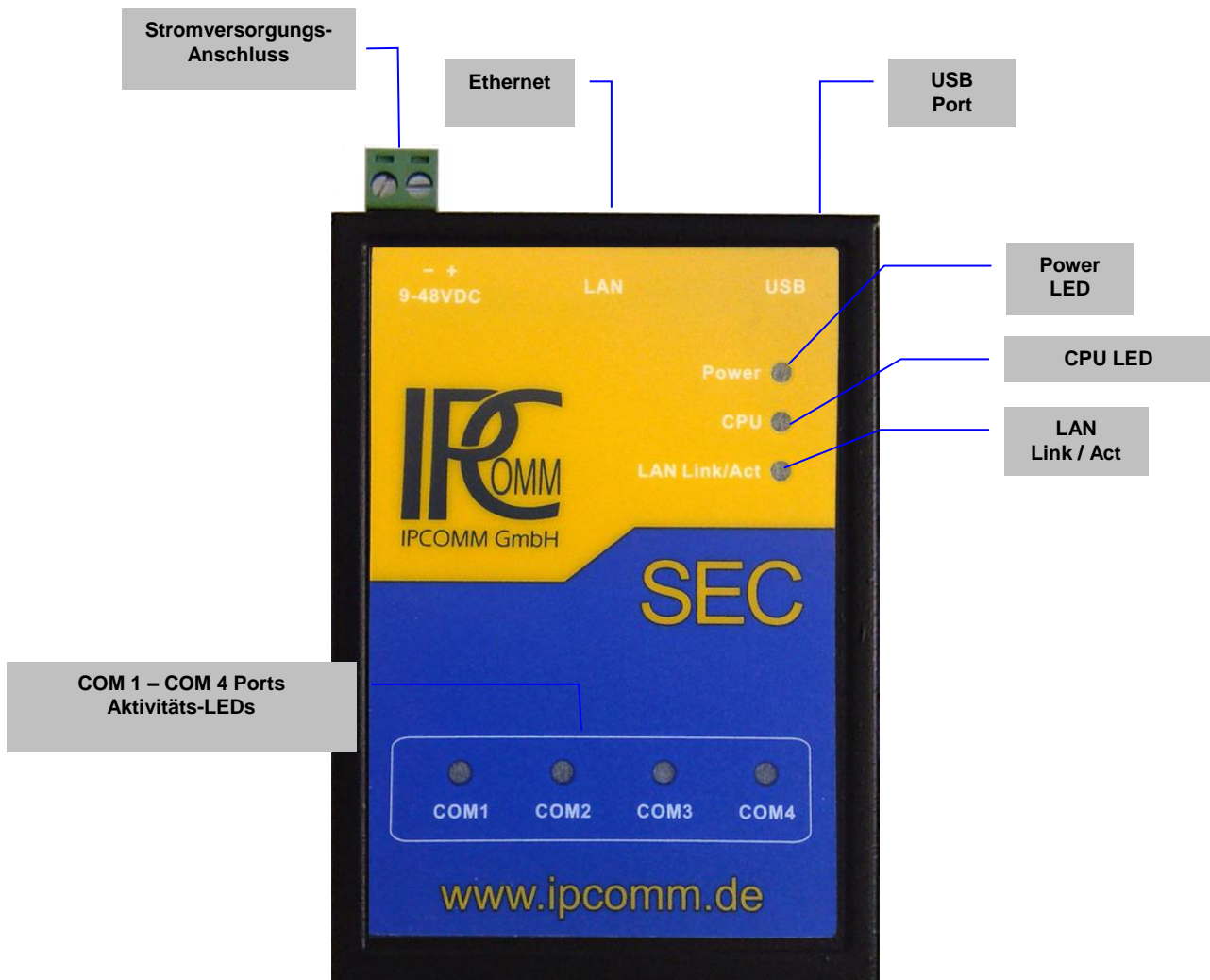
Abbildung 1: SEC2 Vorderansicht
