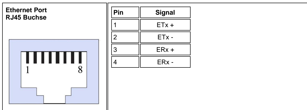
Abbildung 7: Pin-Belegung der Ethernet RJ45 Schnittstelle
