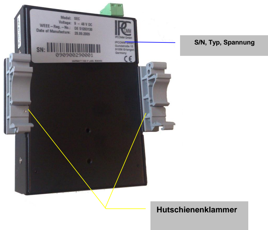
Abbildung 4: SEC2 Rückansicht
