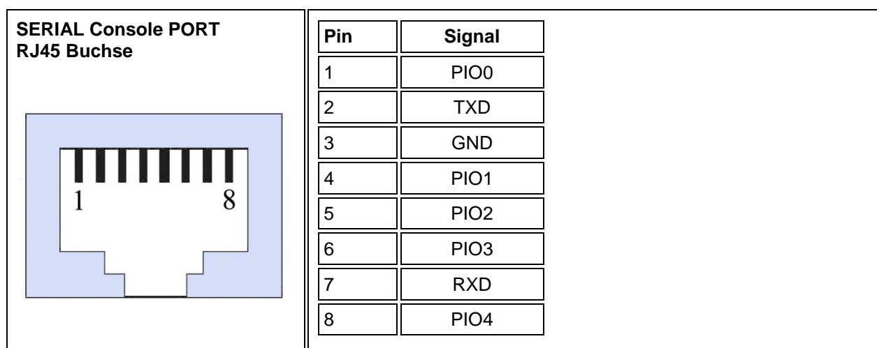
Abbildung 8: Pin-Belegung der RJ45 Schnittstelle als lokale Konsolenverbindung
