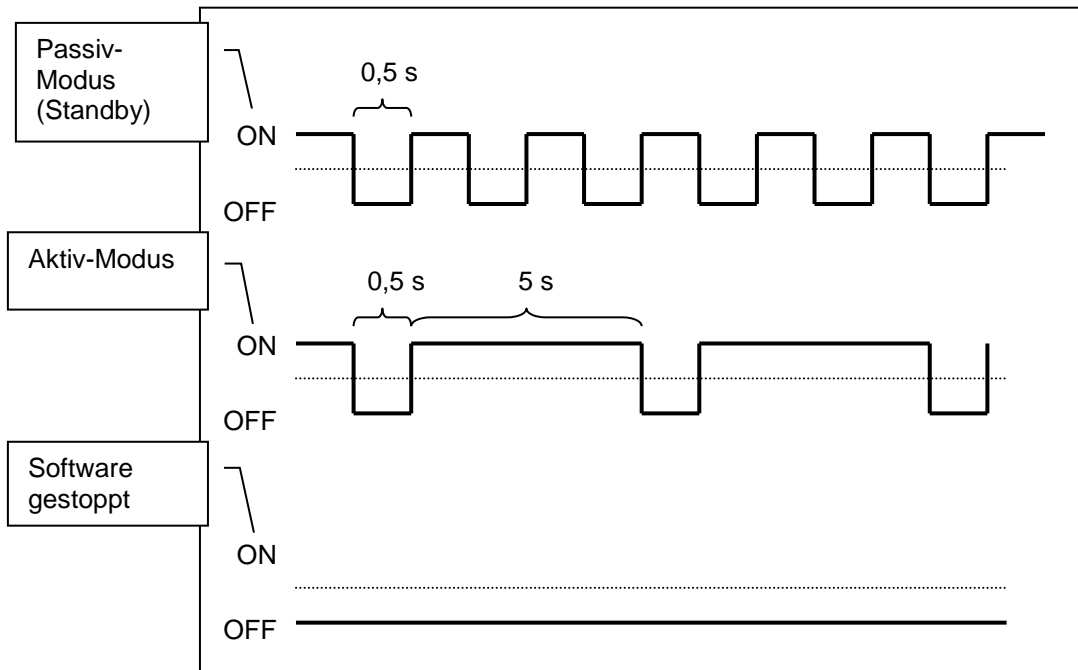
Abbildung 11: CPU-LED Anzeige
