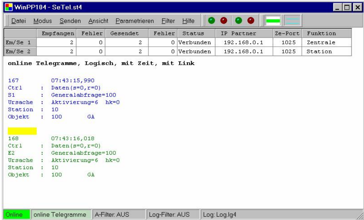
Abb. 1 WinPP104, Online Telegrammanzeige
