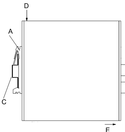
Abb. 2.3.3: Demontage
