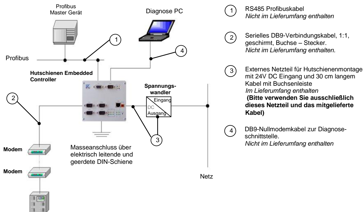
Abb. 2.4: Elektrische Installation - Schaltschema
