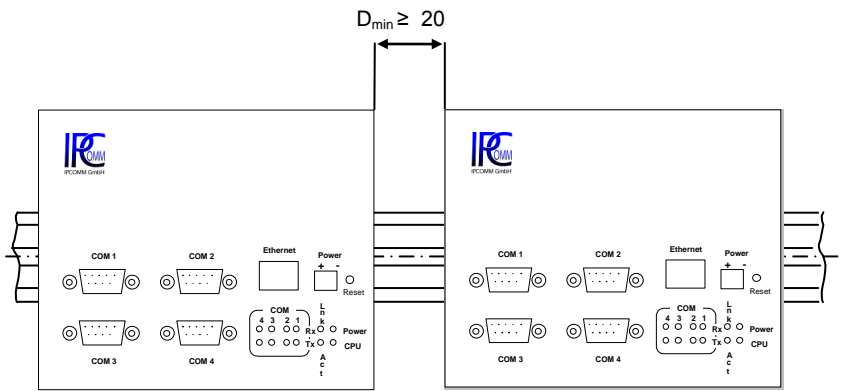
Abb. 2.3.1: Anordnung
