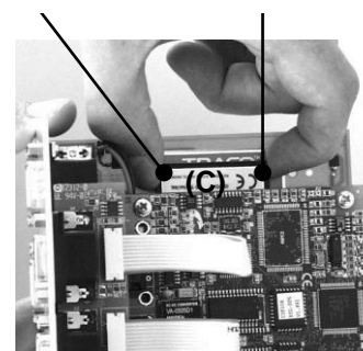
Abb. 2.5.3 Herausziehen der CompactFlash (C)
