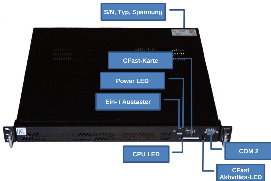
Abbildung 1: IPC191V5 Vorderansicht
