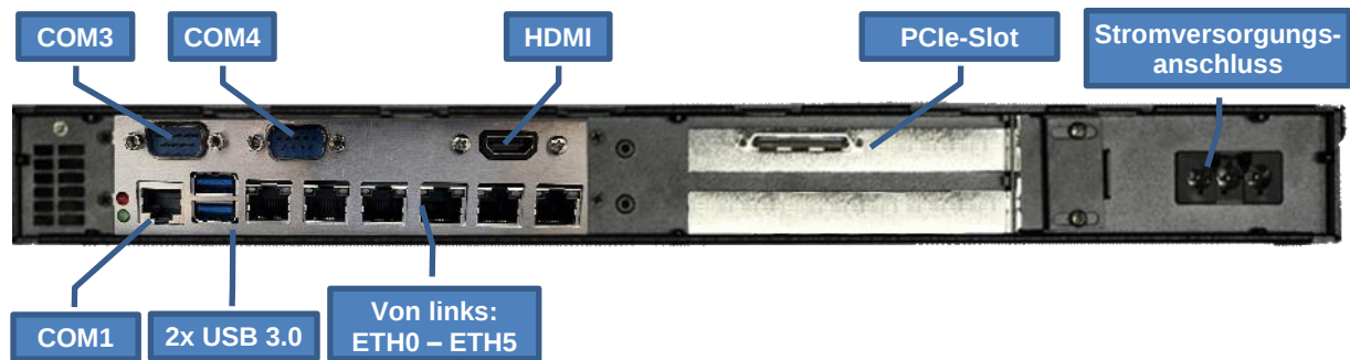
Abbildung 2: Schnittstellenübersicht
