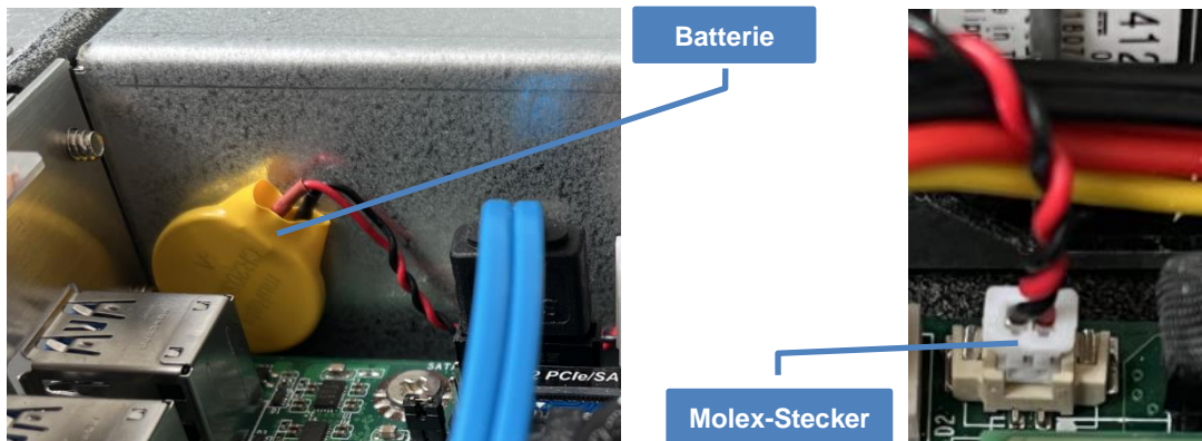
Abbildung 8: Batterie
