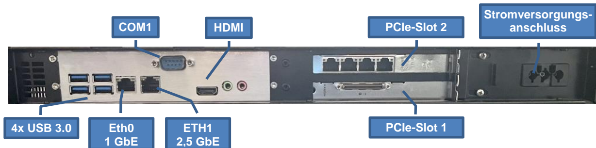
Abbildung 2: Schnittstellenübersicht
