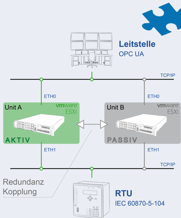
Beispiel für eine Ethernet-basierte Redundanzkopplung.
