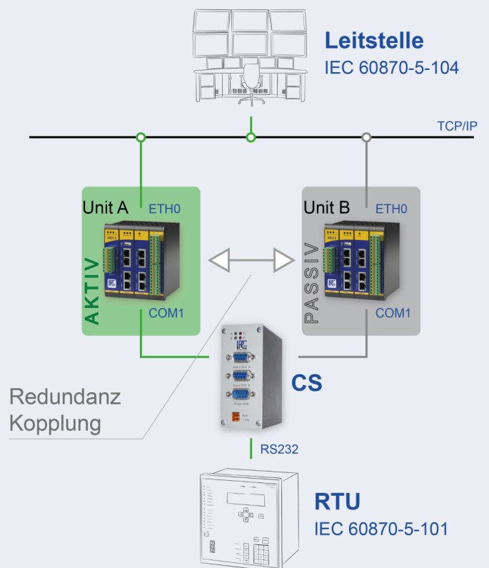
Beispiel einer redundanten Lösung mit ipRoute .
